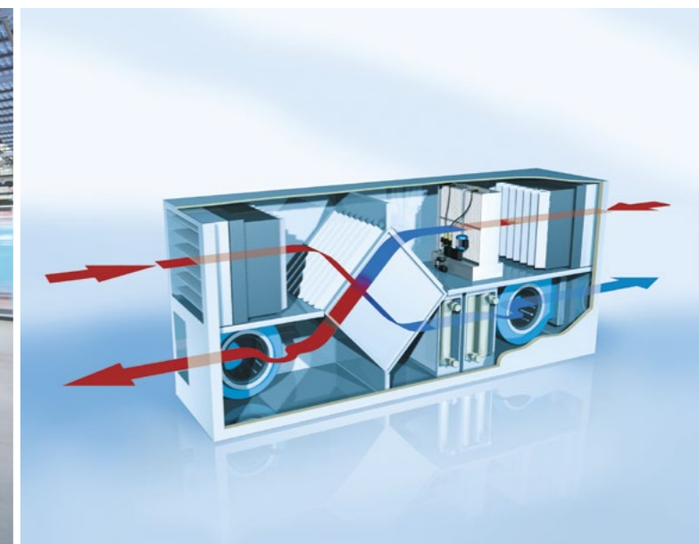
Raffrescamento evaporativo indiretto con Condaire ME
