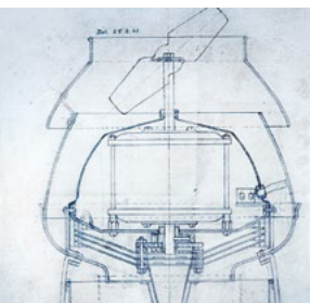
Nebulizzatore rotativo Defensor del 1948
